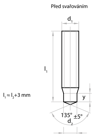
Redukovaný závitový čep RD
